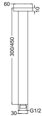
NR504300MB / NR504450MB
